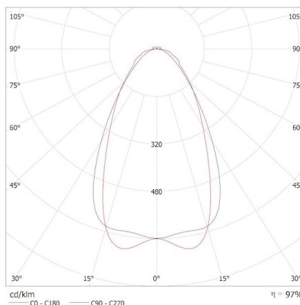
KANLUX S.A. (kat 38391 + 38394) LTL 38W-114-CCT-B 4000K + LENS S 60D / Krzywa rozsyłu światła (biegunowo)
