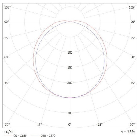
KANLUX S.A. (kat 39501) NOBEN M42W-150-CCT 34W / Krzywa rozsyłu światła (biegunowo)
