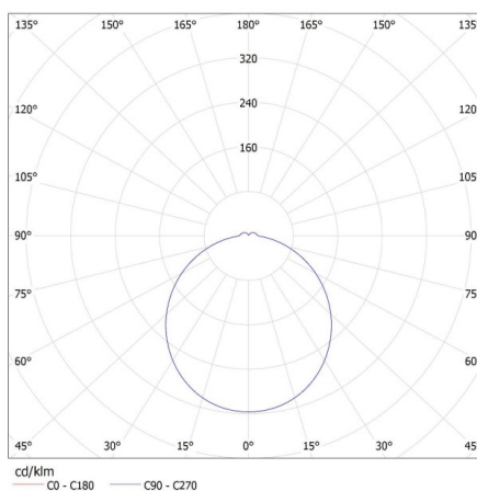
KANLUX S.A. (kat 26985) VARSO HI 36W-NW-O-SE / LDC (Polar)
