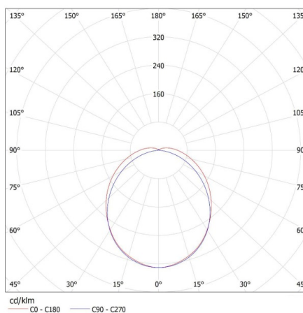
KANLUX S.A. (kat 28686) FT1500 66W-840-RYF / LDC (Polar)
