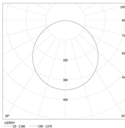
KANLUX S.A. (kat 28950) KANTI V2LED 12W-NW-W / LDC (Polar)
