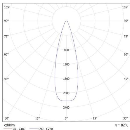
KANLUX S.A. (kat 35654) BTL 28W-930-W 15deg / LDC (Polar)
