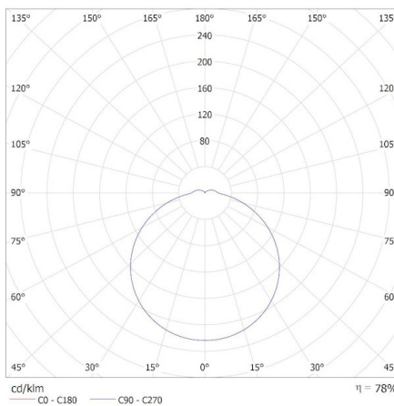
KANLUX S.A. (kat 37292) IPER LED 26W-NW-O / Krzywa rozsyłu światła (biegunowo)
