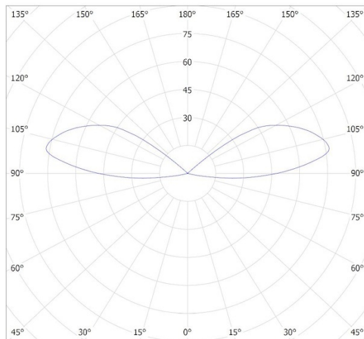
KANLUX S.A. (kat 39184) REFAZI EL 6W-A-O-GR / Krzywa rozsyłu światła (biegunowo)
