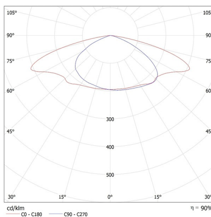
KANLUX S.A. (kat 39289) PRO-S S 10W-ZH NW / Krzywa rozsyłu światła (biegunowo)
