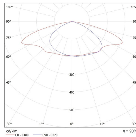
KANLUX S.A. (kat 39295) PRO-S S 40W-ZH NW / Krzywa rozsytu światła (biegunowo)
