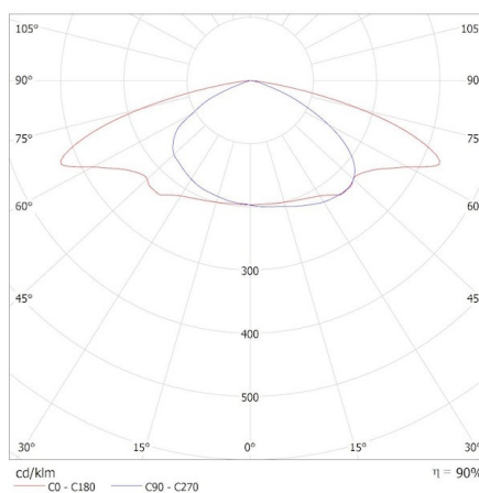
KANLUX S.A. (kat 39298) PRO-S S 55W-ZH NW / Krzywa rozsyłu światła (biegunowo)
