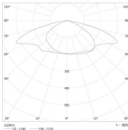
KANLUX S.A. (kat 39299) PRO-S S 60W-ZH NW / Krzywa rozsytu światła (biegunowo)
