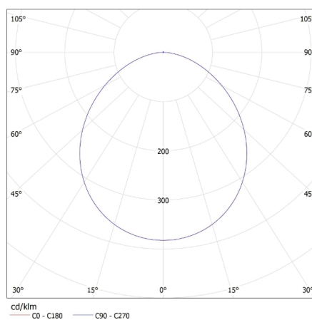
KANLUX S.A. (kat 22706) TOMI LED7W MR16-WW / LDC (Polar)
