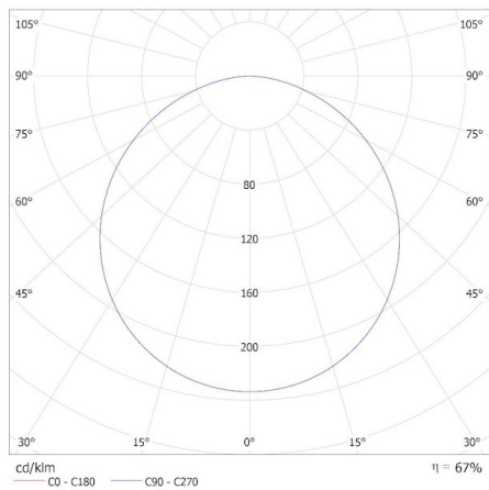
KANLUX S.A. (kat 24606) ERGA PIR 17W CCT-W / Krzywa rozsytu światła (biegunowo)
