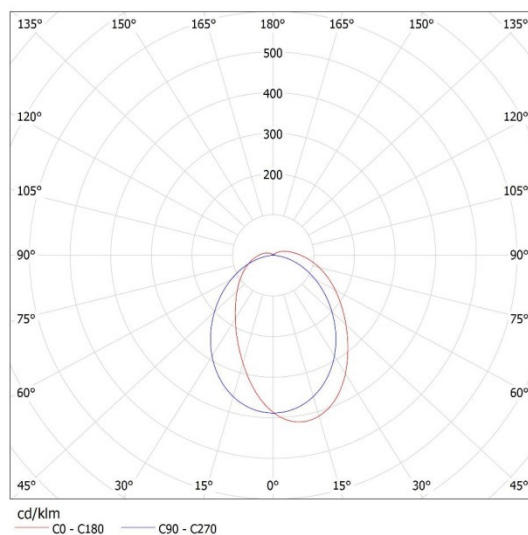
KANLUX S.A. (kat 28634) FT1200 37W-840-ASY / LDC (Polar)
