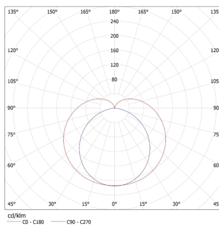
KANLUX S.A. (kat 29213) MERA LED 20W NW / LDC (Polar)
