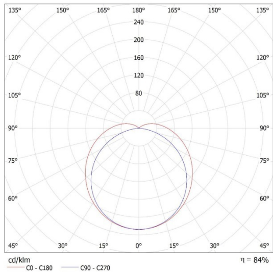
MILED0 (kat 31410) DIGHT LED 18W-NW / LDC (Polar)
