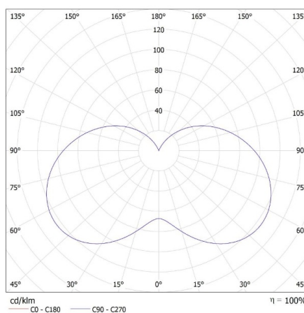
KANLUX S.A. (kat 33729) IQ-LED C37E14 4,2W-NW / LDC (Polar)
