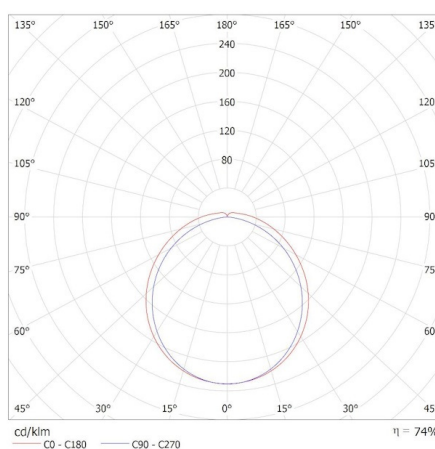
KANLUX S.A. (kat 33892) MEBA LED 20W IP54 NW / Krzywa rozsyłu światła (biegunowo)
