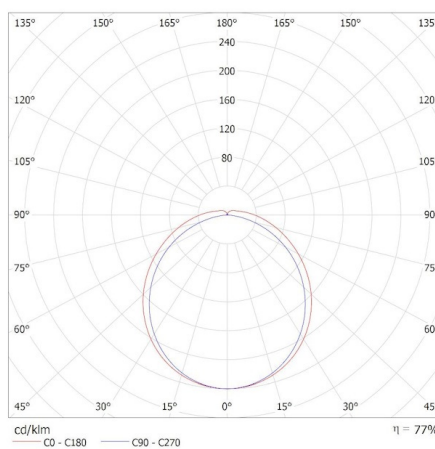
KANLUX S.A. (kat 33893) MEBA LED 40W IP54 NW / Krzywa rozsyłu światła (biegunowo)
