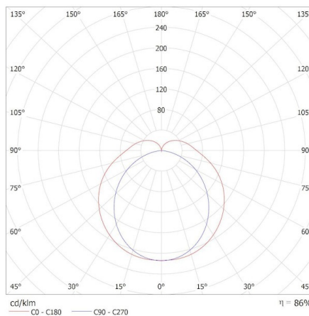
KANLUX S.A. (kat 36665) AKVO IP44 23W-NW-W / Krzywa rozsyłu światła (biegunowo)
