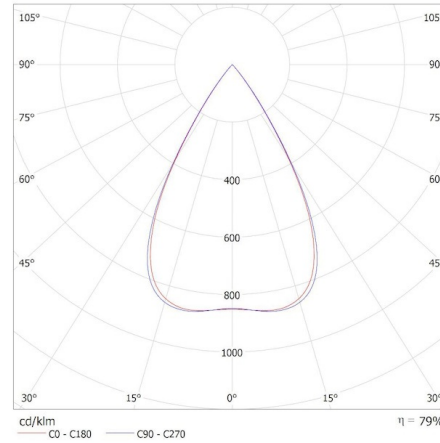
KANLUX S.A. (kat 37054) HR-LM-WN-B-PT / Krzywa rozsyłu światła (biegunowo)
