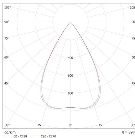
KANLUX S.A. (kat 37114) HR-LH-WW-W-RM / Krzywa rozsytu światła (biegunowo)
