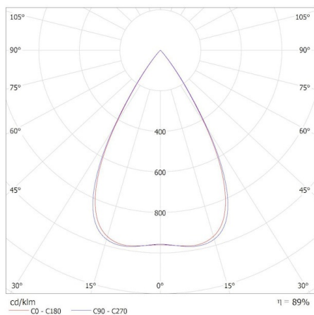
KANLUX S.A. (kat 37139) HR-MH-NW-W-RM / Krzywa rozsytu światła (biegunowo)
