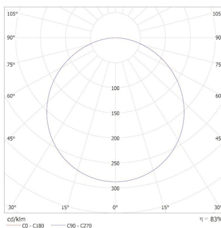
KANLUX S.A. (kat 37170) BLINGO 34W 3740 60WW / Krzywa rozsyłu światła (biegunowo)
