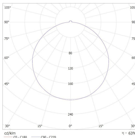
KANLUX S.A. (kat 37318) NIFU LED17,8W NW W_W / Krzywa rozsyłu światła (biegunowo)
