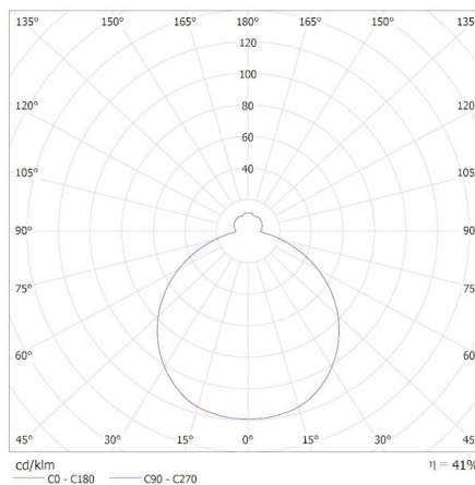
KANLUX S.A. (kat 37324) SOLN LED 17,5W NW B/G / Krzywa rozsyłu światła (biegunowo)
