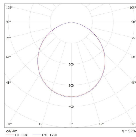
KANLUX S.A. (kat 38123) DAXA-S 5W CCTDIM W / Krzywa rozsyłu światła (biegunowo)
