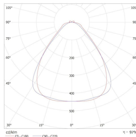
KANLUX S.A. (kat 38391) LTL 38W-114-CCT-B 3000K / Krzywa rozsyłu światła (biegunowo)
