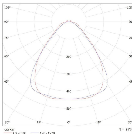
KANLUX S.A. (kat 38392) LTL 38W-114-CCT-ADJ-W 3000K / Krzywa rozsyłu światła (biegunowo)
