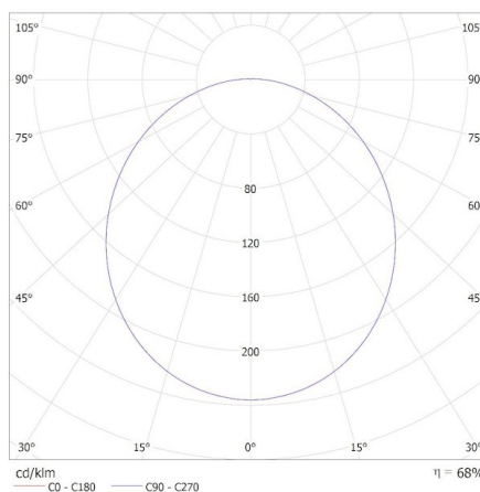
KANLUX S.A. (kat 38775) BENO 12-18W CCT-L-SEW 12W / Krzywa rozsyłu światła (biegunowo)
