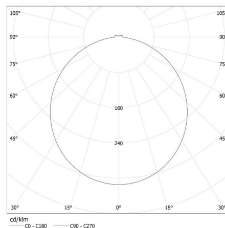
KANLUX S.A. (kat 26771) AVAR 6060 40W-CW / LDC (Polar)
