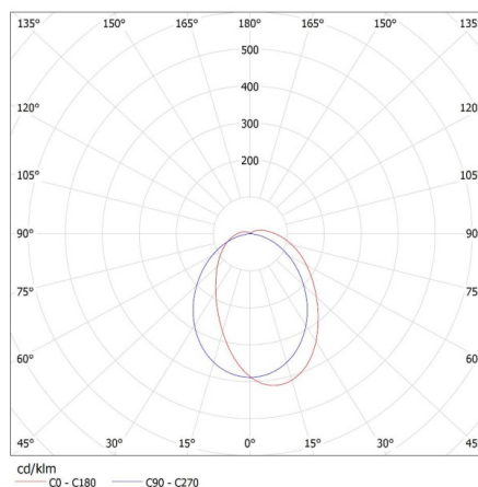
KANLUX S.A. (kat 28853) FT1200 28W-840-ASY / LDC (Polar)
