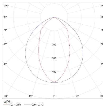
MILED0 (kat 31058) RSTR N 236/4LED/NT i GLASSv2 / LDC (Polar)
