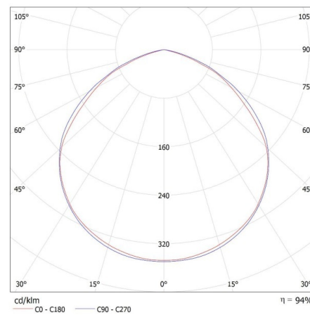
MILEDO (kat 31392) GRUN NV LED-30-B / LDC (Polar) Luminaire: MILEDO (kat 31392) GRUN NV LED-30-B Lamps: 1 x GRUN NV LED-30-B
