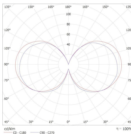
KANLUX S.A. (kat 36245) XLED EX A60 5W-WW / Krzywa rozsyłu światła (biegunowo)
