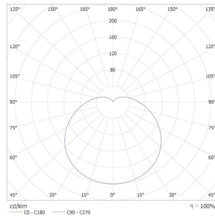
KANLUX S.A. (kat 36672) IQ-LED A60 3,4W-CW / Krzywa rozsytu światła (biegunowo)
