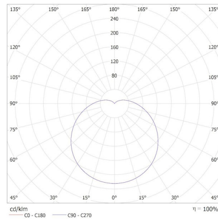
KANLUX S.A. (kat 36690) IQ-LED G45E14 3,4W-CW / Krzywa rozsytu światła (biegunowo)
