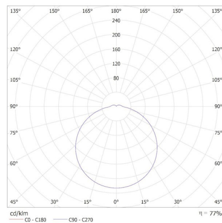
KANLUX S.A. (kat 37301) IPER LED 35W-NW-O-SE / Krzywa rozsyłu światła (biegunowo)
