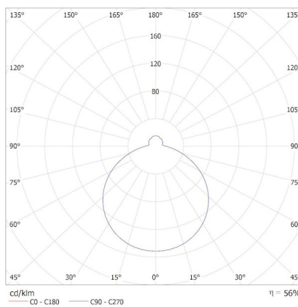
KANLUX S.A. (kat 37330) ARVOS LED 37W CCT B / Krzywa rozsyłu światła (biegunowo)
