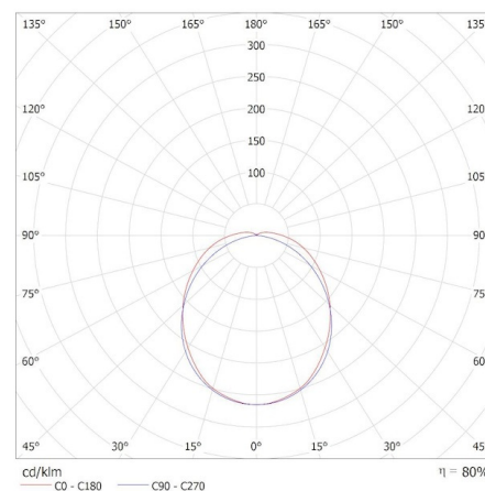
KANLUX S.A. (kat 38465) MAH MAX 48W 15 NW RYF / Krzywa rozsyłu światła (biegunowo)
