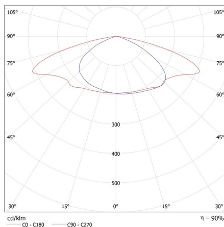
KANLUX S.A. (kat 39295) PRO-S S 40W-ZH NW / Krzywa rozsyłu światła (biegunowo)
